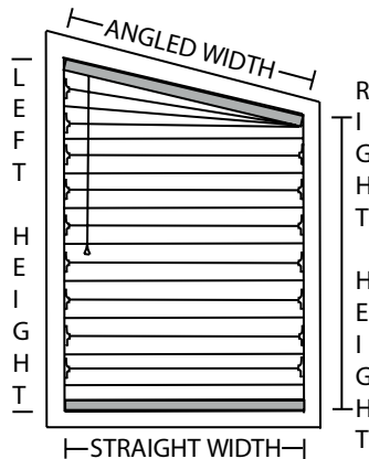
Angled Top
